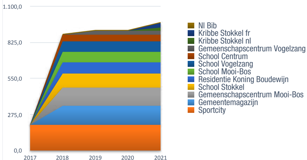
Evolutie van de geïnstalleerde fotovoltaïsche capaciteit
